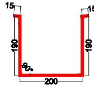
Box Gutter 1 Code : BG(1)610
